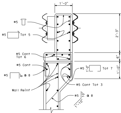
SECTION D-D
